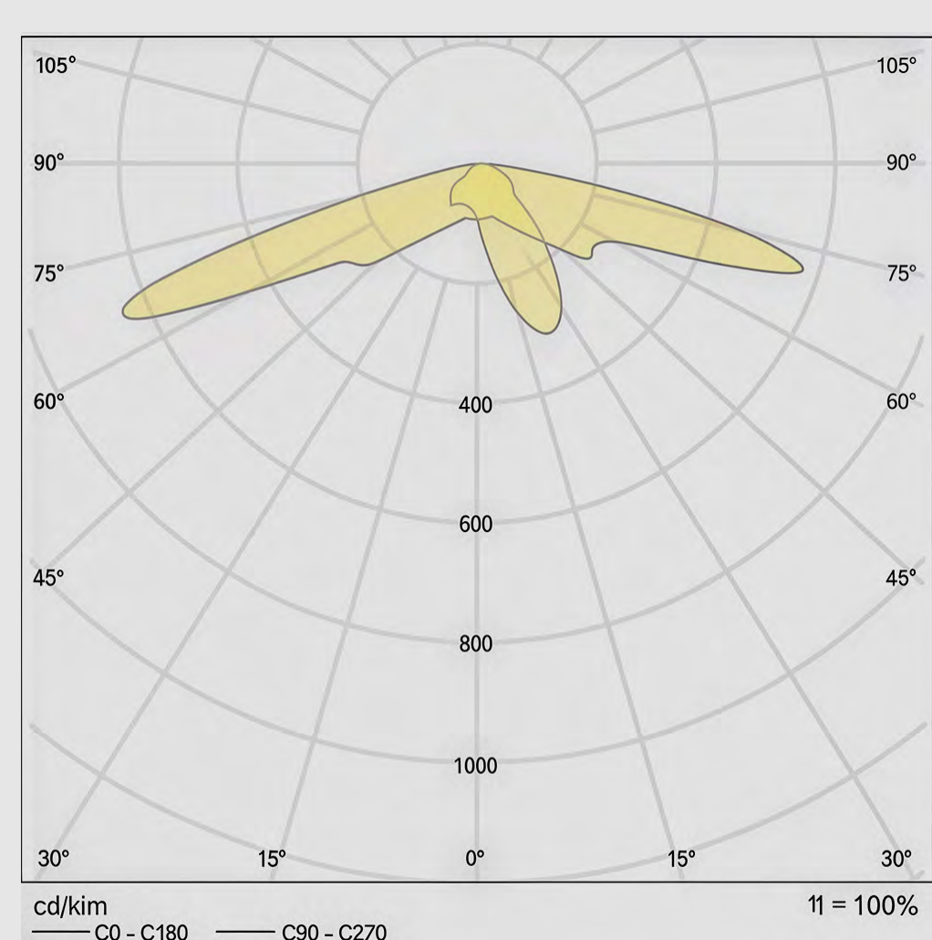
Vialed 70W Tipo II M
