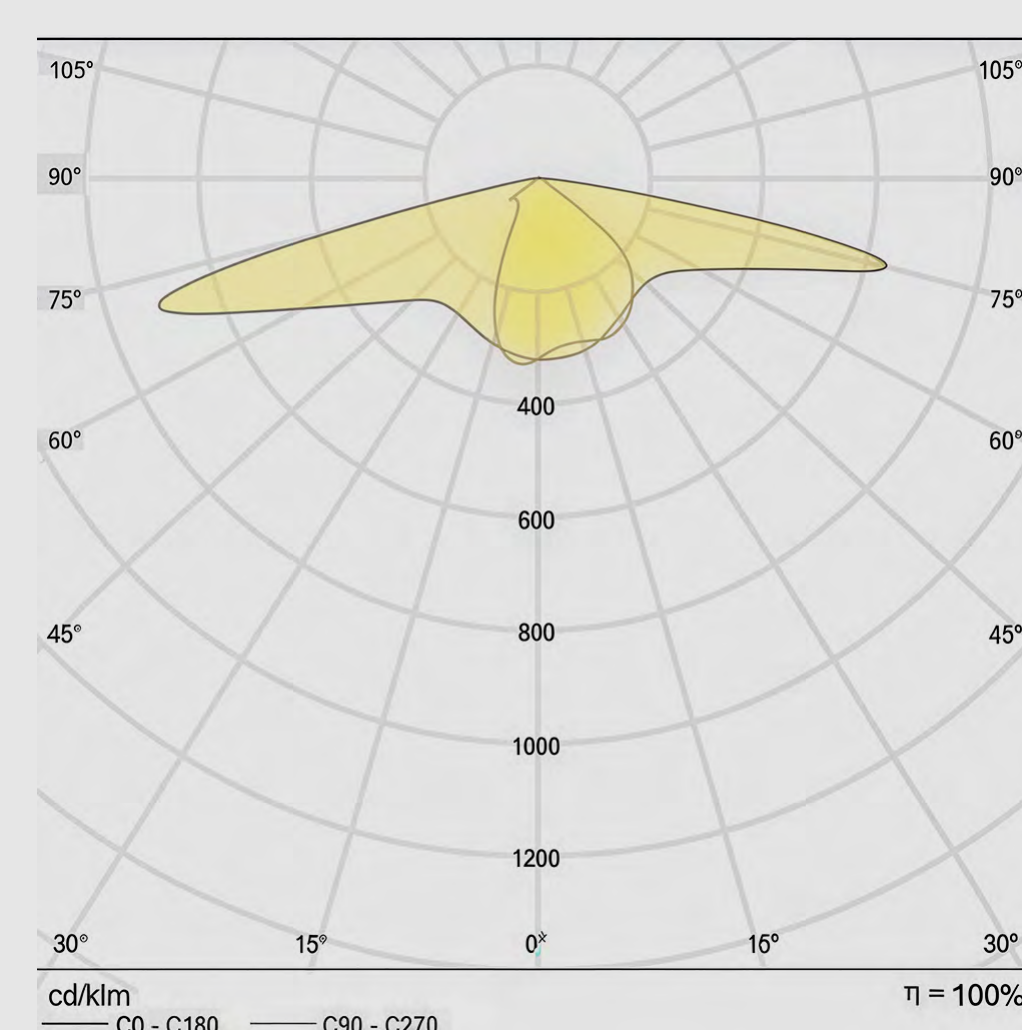
Vialed 130W Tipo II M
