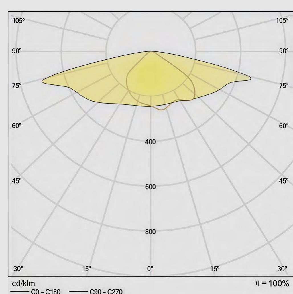
Vialed 50W Tipo II M
