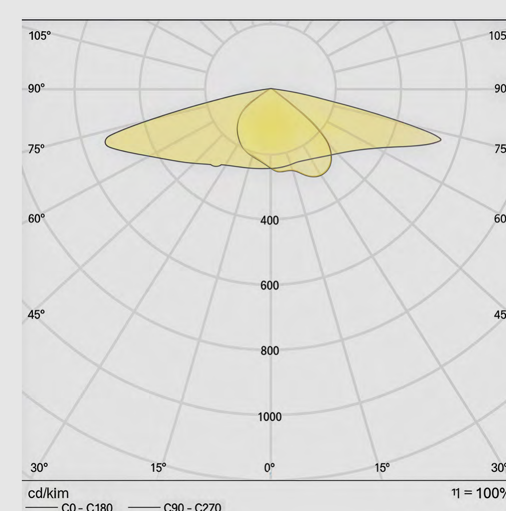
Vialed 160W Tipo II M
