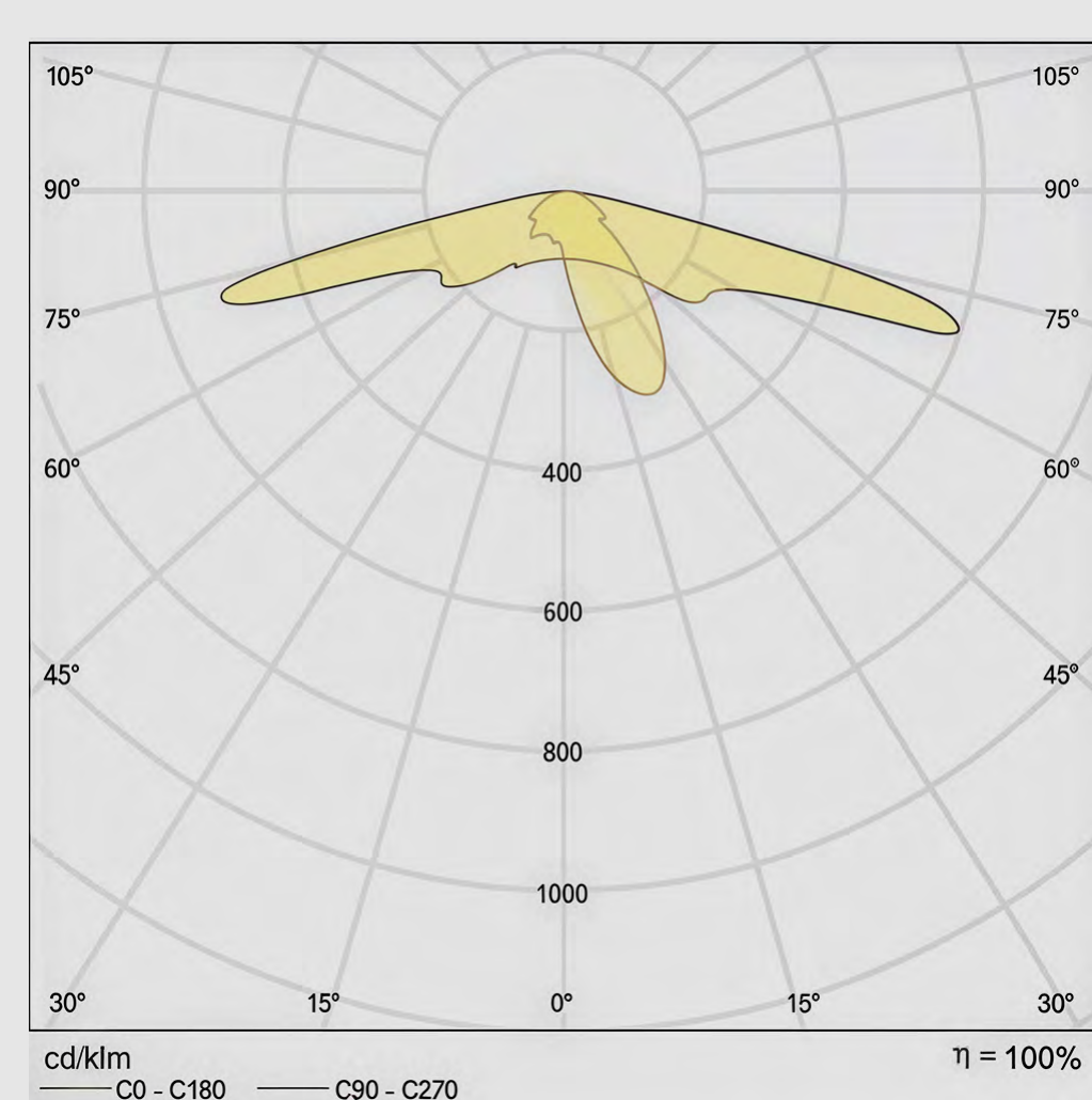
Vialed 100W Tipo II M
