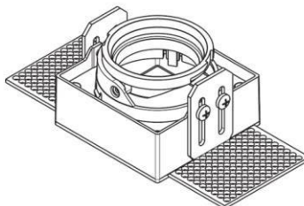
Cuadrado empotrado Trimless
