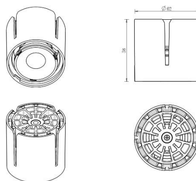
Dimensiones de CO1030
